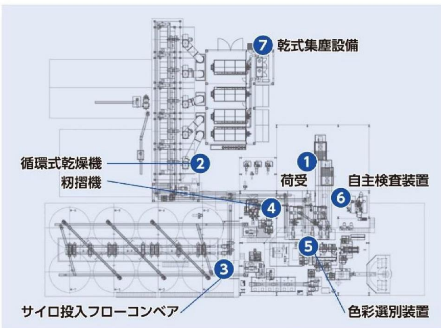
【南部カントリーエレベーター平面図】
