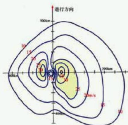
気象庁(1961):伊勢湾台風調査報告、気象庁技術報告第7号。 伊勢湾台風の進路と風速の分布
